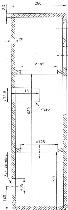
CUT A-A
